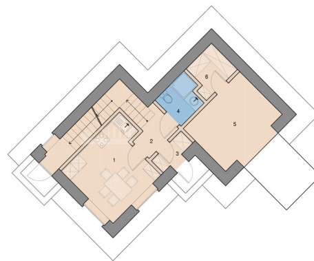
Гостевой дом 1-й этаж
