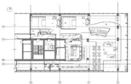
ПЛАН 59 ЭТАЖА
